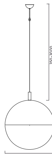
Vajerpendel/Wire pendant
