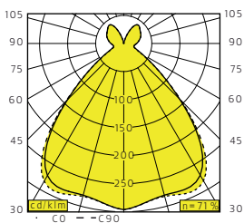
Metallhalogen/Metal halide
