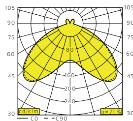
Kompaktlysörör/Compact fluorescent
