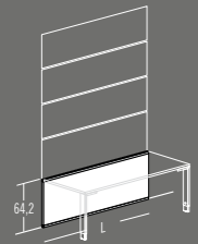
SEBT42 L 80÷120 SEBT44 L 120÷140 SEBT46 L 140÷160 SEBT48 L 160÷180 SEBT50 L 180÷200 SEBT54 L 200÷240 SEBT58 L 240÷280
