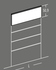
SEBS72 L 80÷120 SEBS74 L 120÷140 SEBS76 L 140÷160 SEBS78 L 160÷180 SEBS80 L 180÷200 SEBS84 L 200÷240 SEBS88 L 240÷280
