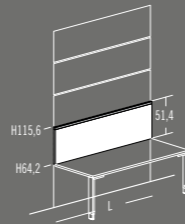
SEBI72 L 80÷120 SEBI74 L 120÷140 SEBI76 L 140÷160 SEBI78 L 160÷180 SEBI80 L 180÷200 SEBI84 L 200÷240 SEBI88 L 240÷280
