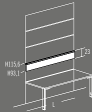
SEBI12 L 80÷120 SEBI14 L 120÷140 SEBI16 L 140÷160 SEBI18 L 160÷180 SEBI20 L 180÷200 SEBI24 L 200÷240 SEBI28 L 240÷280
