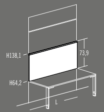
SEBI112 L 80÷120 SEBI114 L 120÷140 SEBI116 L 140÷160 SEBI118 L 160÷180 SEBI120 L 180÷200 SEBI124 L 200÷240 SEBI128 L 240÷280
