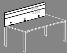
SE0702 L120 P1,8 H48 SE0704 L140 P1,8 H48 SE0706 L160 P1,8 H48 SE0708 L180 P1,8 H48 SE0710 L200 P1,8 H48
