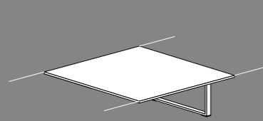
SQ1636 L160 P160 H72 SQ1638 L180 P160 H72
