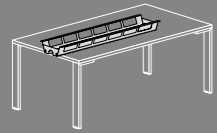
SE9212 mod.120 L74 P25,5 H11 SE9214 mod.140 L94 P25,5 H11 SE9216 mod.160 L114 P25,5 H11 SE9218 mod.180 L134 P25,5 H11 SE9220 mod.200 L154 P25,5 H11
