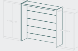
CXBI19SC L164 P55,2 H202 CXBI23SC L204 P55,2 H202
