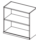
AGHNO-CG84 cm. 90 L 45 P 84 H in. 35,4 W 17,7 D 33,1 H
