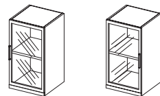
AGHNO-CPV84/45DS cm. 45 L 45 P 84 H in. 17,7 W 17,7 D 33,1 H
